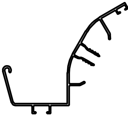
Tagrende profil
